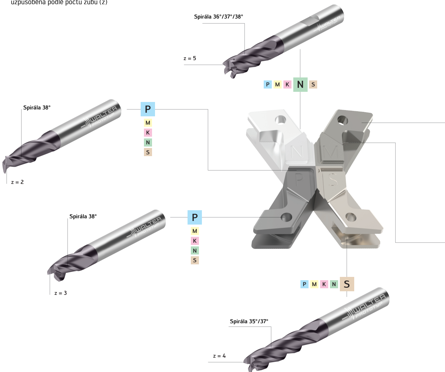
Fréza ze slinutého karbidu Xill-tec® MC230 Advance
