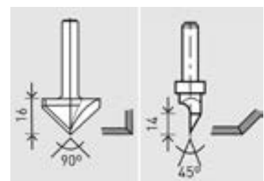
Fréza na sádrokarton 90° (objednací č. 491001) Fréza na sádrokarton 45° (objednací č. 491000)
