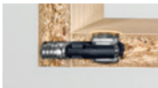
Úhlový svorník – pro spojení DOMINO/DOMINO
